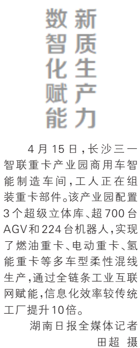
4月15日，长沙三一智联重卡产业园商用车智能制造车间，工人正在组装重卡部件。该产业园配置3个超级立体库、超700台AGV和224台机器人，实现了燃油重卡、电动重卡、氢能重卡等多车型柔性混线生产，通过全链条工业互联网赋能，信息化效率较传统工厂提升10倍。
