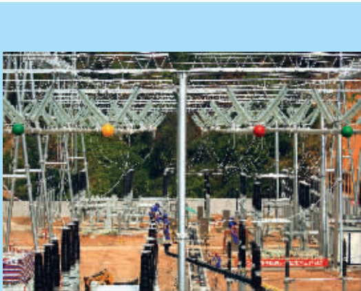
220 千伏会同输变电工程施工现场(邓武摄)
