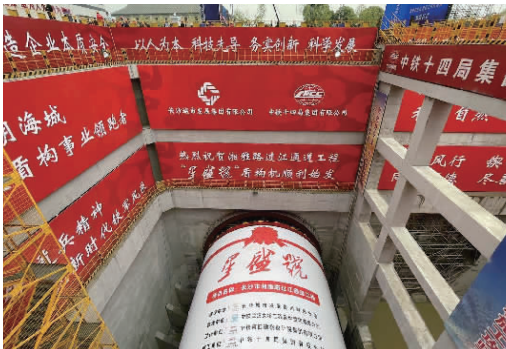
3月30日上午，长沙湘雅路过江通道“星盛号”盾构机始发。记者周可摄
