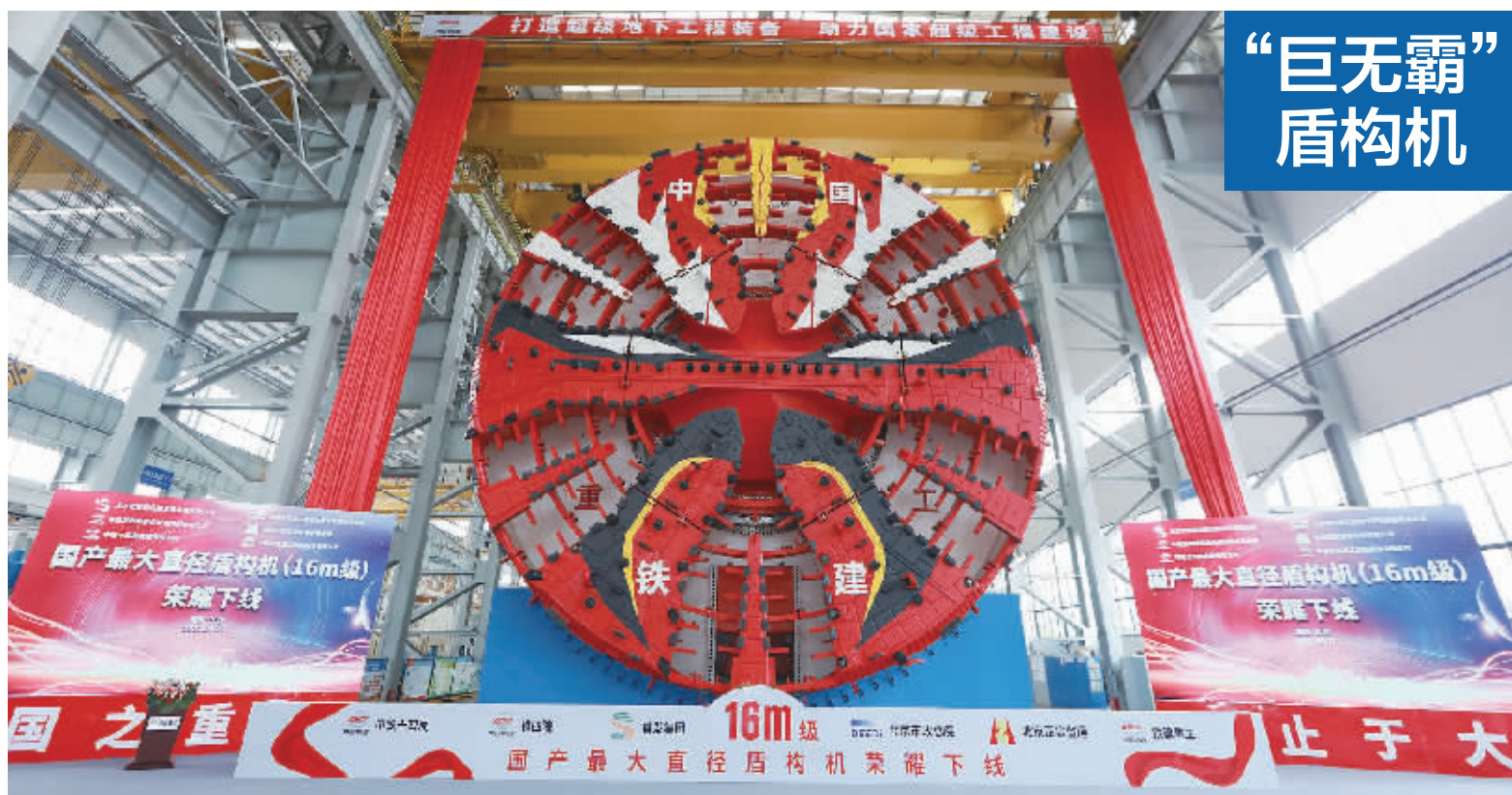
9月27日,一台最大开挖直径达16.07米的超大直径盾构机在中国铁建重工集团长沙第一产业园下线。这台取名“京华号”的“巨无霸”盾构机整机长150米,总重量4300吨,是我国迄今研制的最大直径盾构机。
