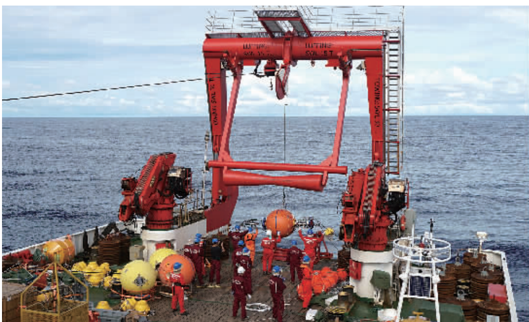
2月7日，我国新一代海洋综合科考船“科学”号在完成2017年西太平洋综合考察航次后，返回青岛西海岸新区的母港。科考队员在本航次成功建成我国首个深海实时科学观测网，西太平洋深海3000米范围内的温度、盐度和洋流等数据实现1小时1次实时传输。 新华社图
