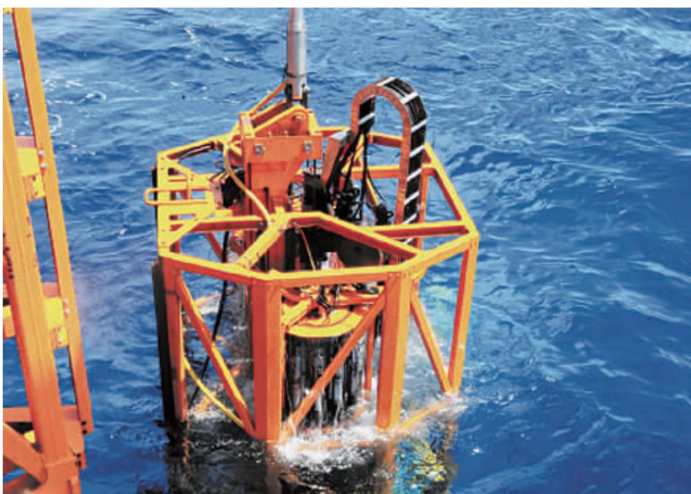
湖南科技大学研制的“海牛”深海钻机,要在3000米深的海底开展作业,离不开深海电缆。
